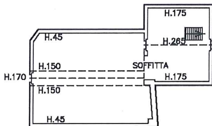
PIANO TERZO (SOTTOTETTO)
